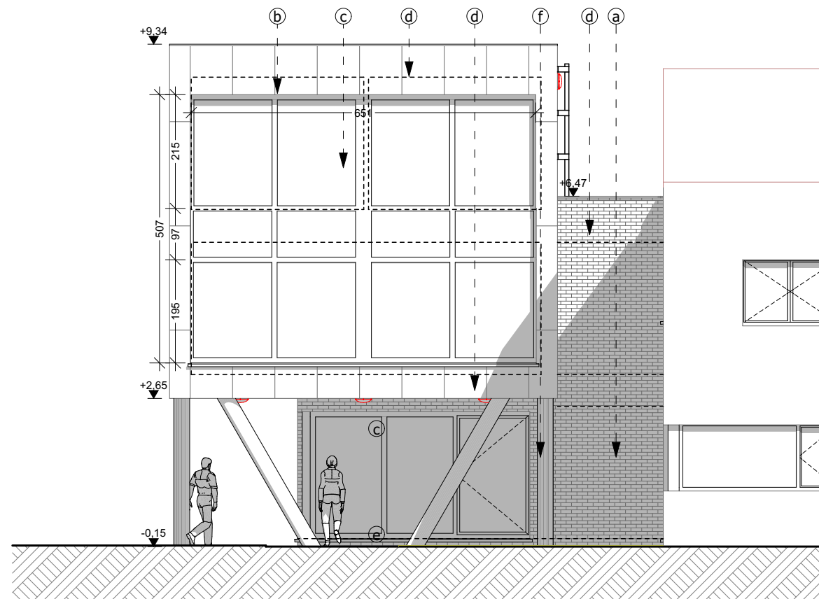
Façade avant - situation projetée - échelle 1/100 ème
