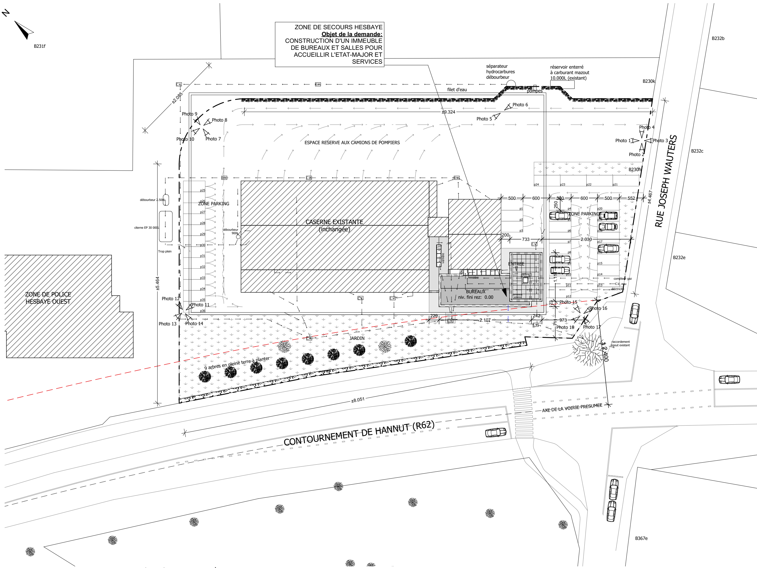
Plan implantation - situation projetée - échelle 1/500 ème
