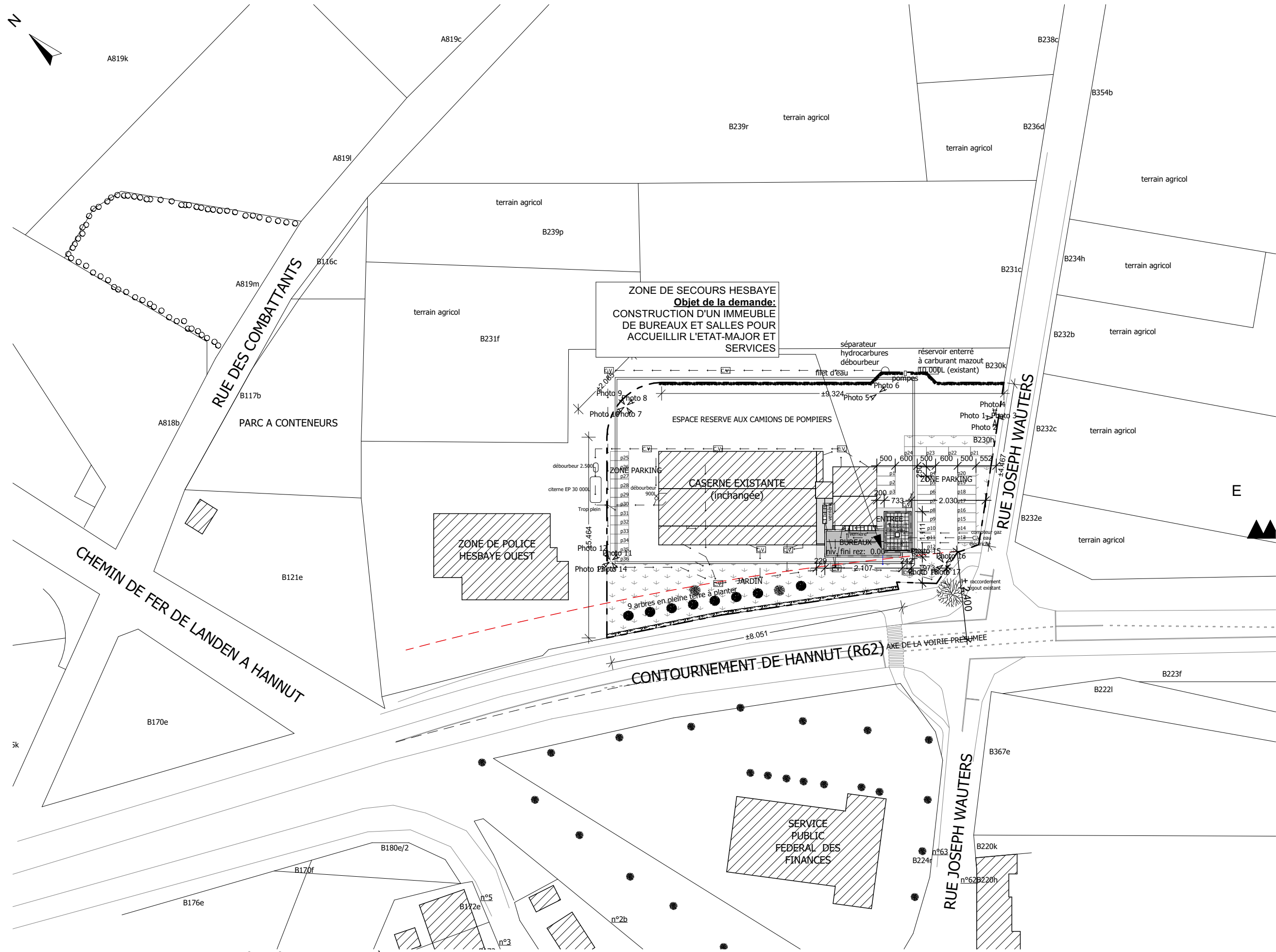
Plan implantation - situation projetée - échelle 1/1.000 ème
