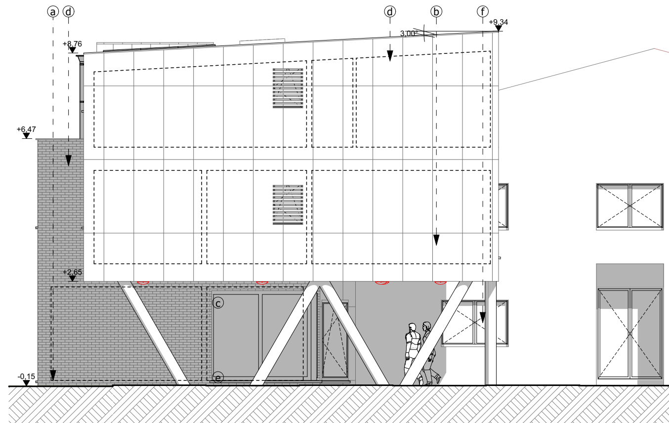
Façade latérale gauche - situation projetée - échelle 1/100 ème
