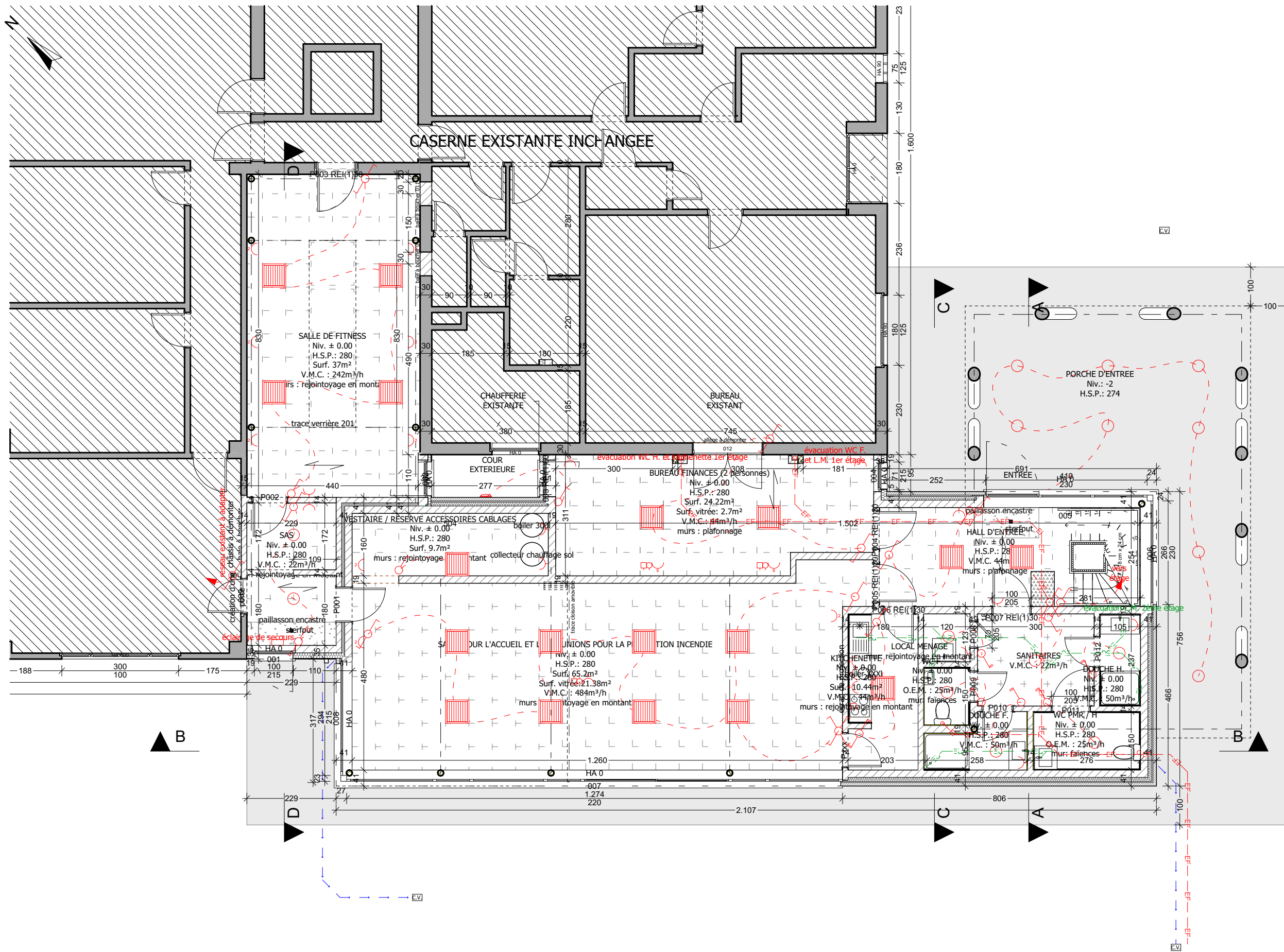
Plan rez-de-chaussée - situation projetée - échelle 1/100 ème
